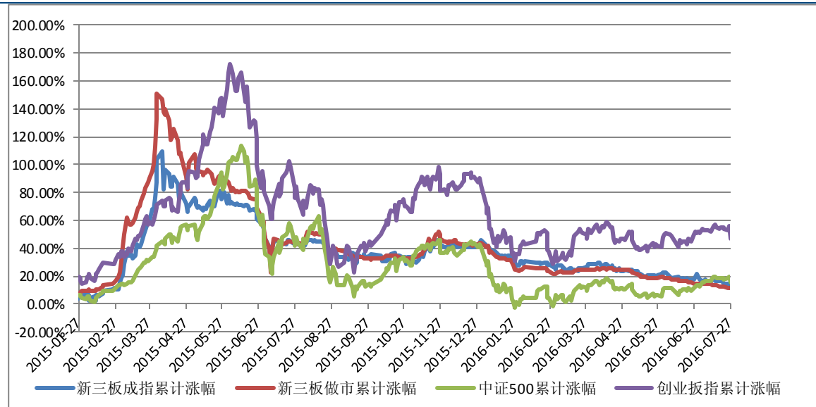
图 1: 新三板成指、新三板做市、中证500、创业板指走势
